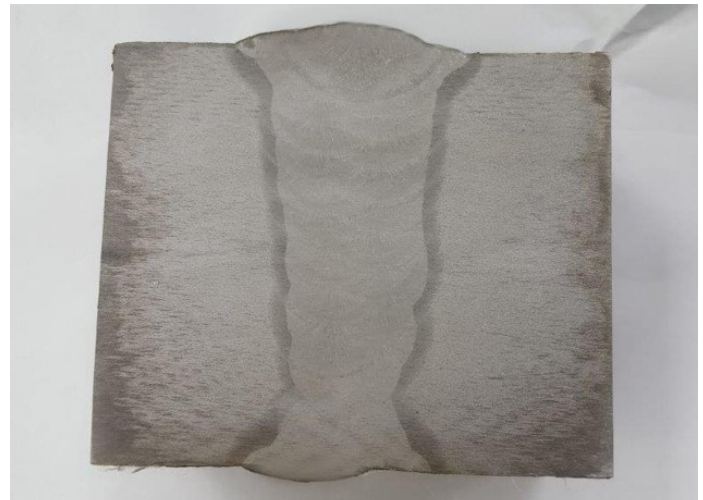
銲道巨觀
